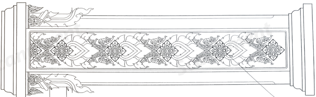
แบบขยายลดดลาย 6 มาตราส่วน 1 : 25
