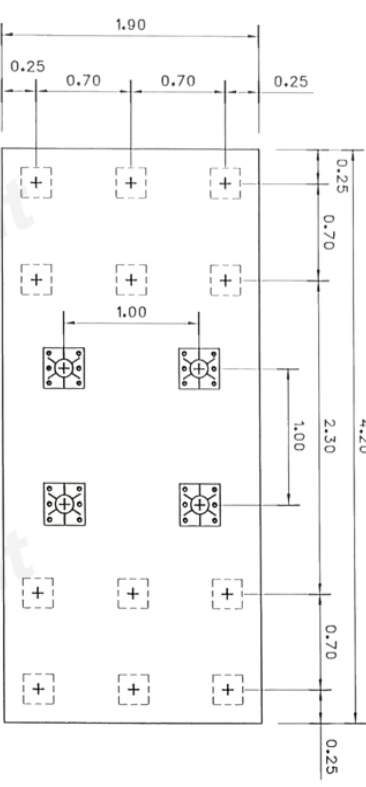
แบบขยายฐานราก F1 1:40 วิศวกรคำนวณ
