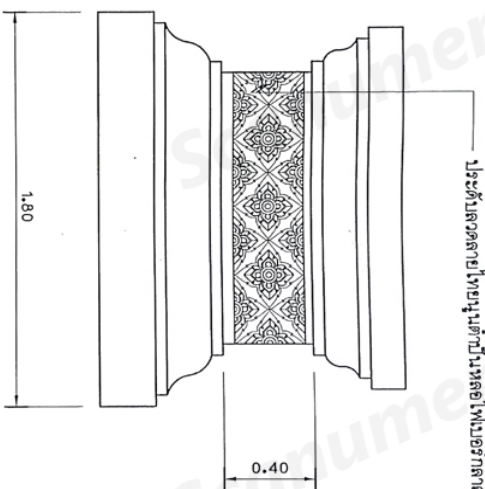
แบบขยายลดดลาย 7 มาตราส่วน 1 : 25
