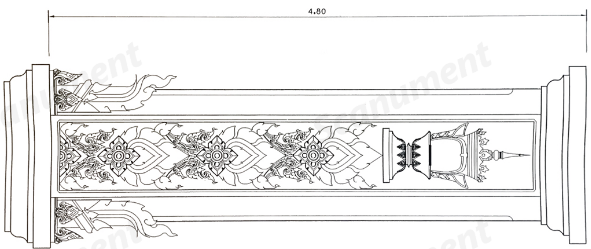
แบบขยายชุดลาย 9 ขนาดตาม 1 : 25
