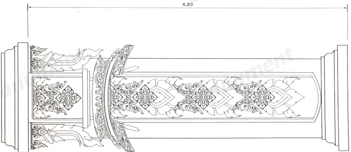
แบบขยายชุดลาย 8 ขนาดตาม 1 : 25
